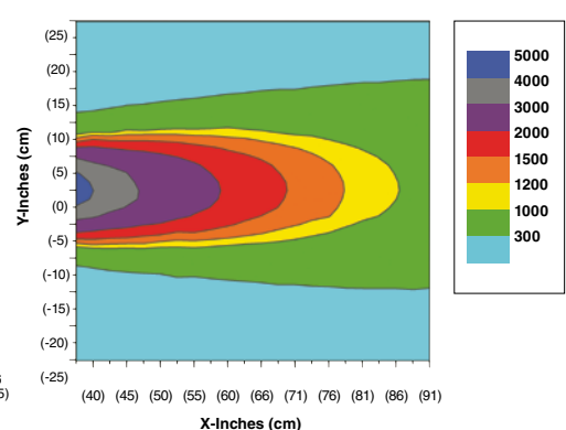
Longitudinal Profile
